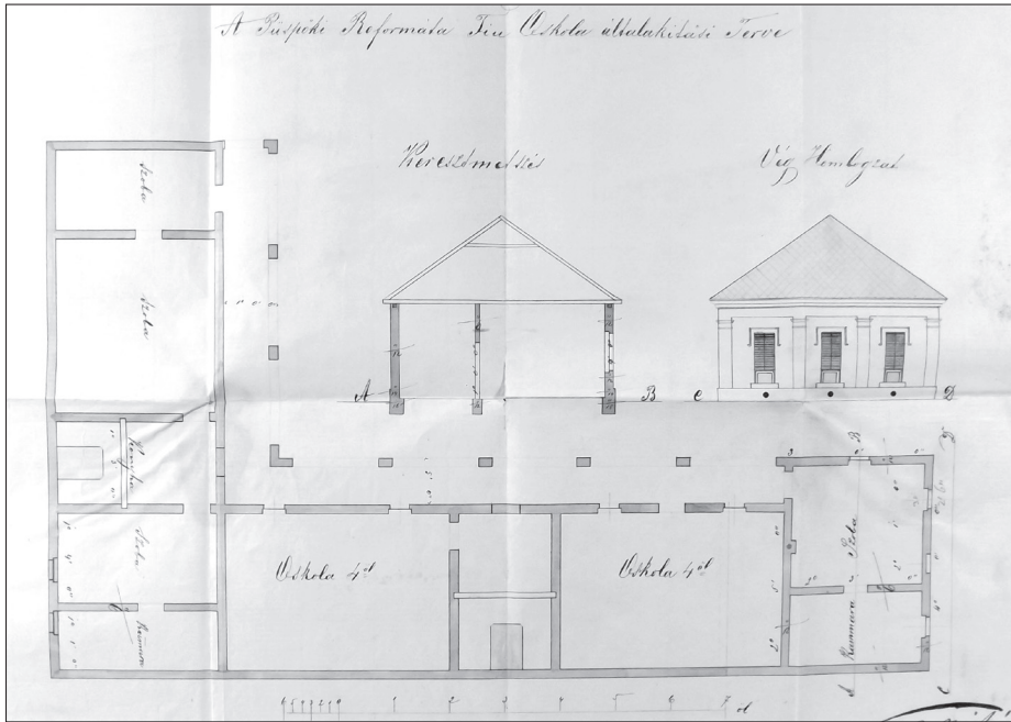
Az 1773-ban épült újabb biharpüspöki fiúiskola átalakítási tervrajza 1867-ből
